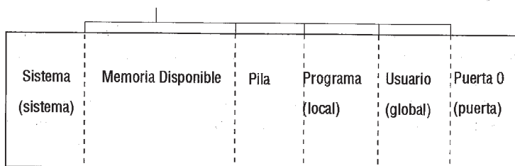
Presentación esquemática de la RAM del sistema en la HP 48
