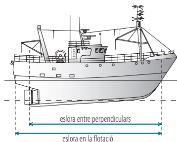
ESLORA
