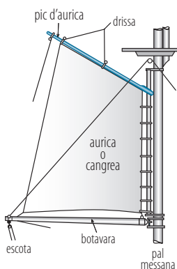
PIC D'AURICA
