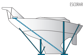
ESCORAR
