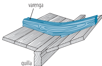
VARENGA
