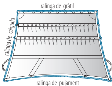
RALINGA
